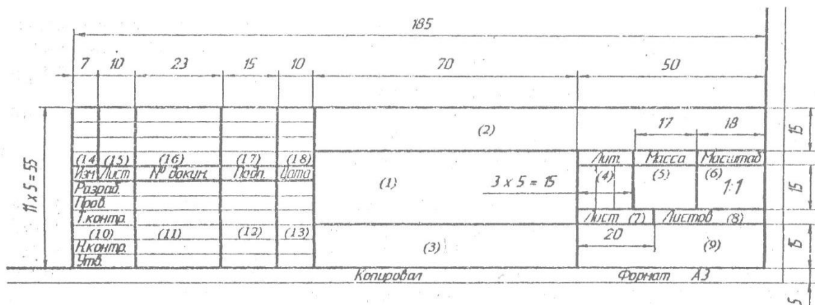
Рисунок 5 – Форма и размеры основной надписи для графического листа в соответствии с ГОСТ 2.104
