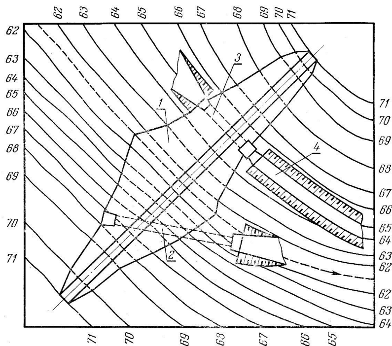
Рисунок 35 - План гидроузла
